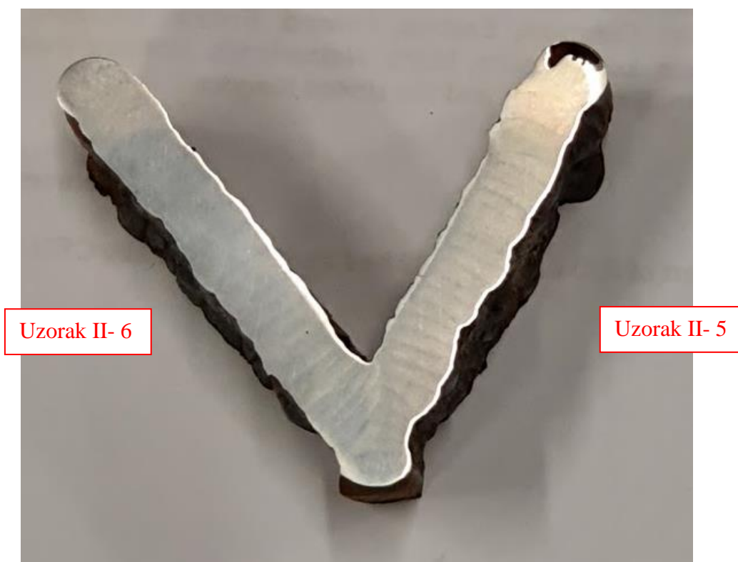
Slika 54. Rezultati nagrizanja površine na uzorak II- desna strana
