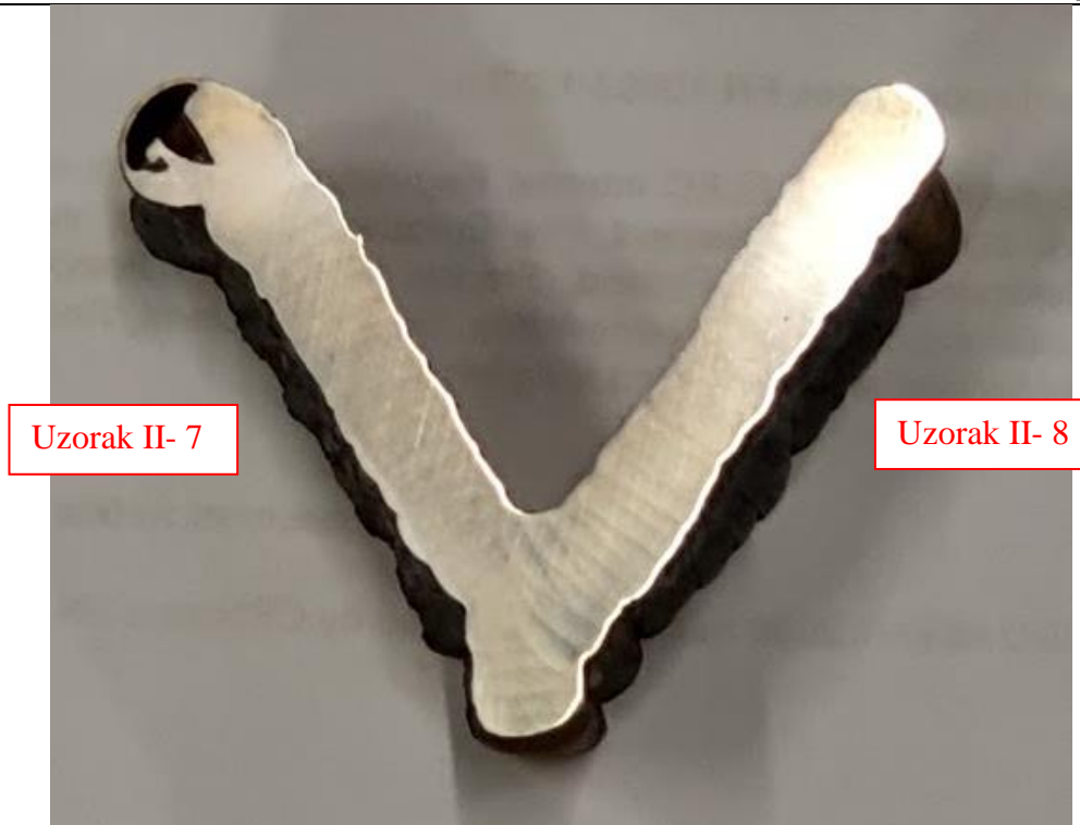
Slika 53. Rezultati nagrizanja površine na uzorak II- lijeva strana
