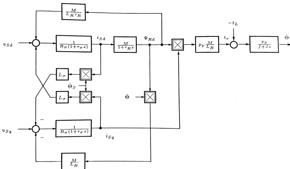
Slika 5.3 Model asinkronog stroja u rotorskom koordinatnom sustavu [10]
