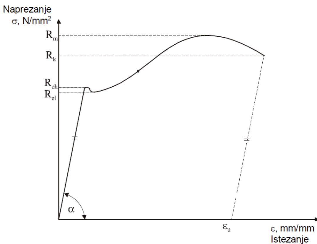
Slika 10. Konvencionalni dijagram naprežanje-istežanje[1]
