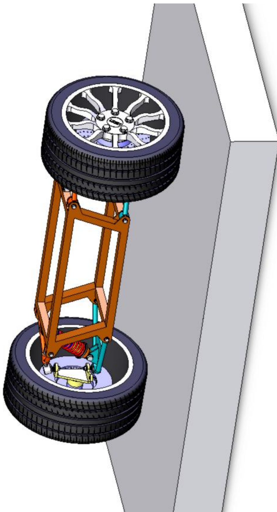
Trodimenzijski model neovisnog ovjesa (Solidworks 2004)
