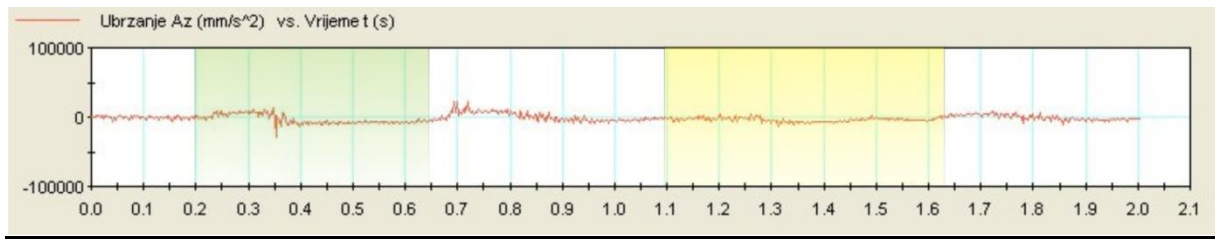
Slika 6.20 Dijagram ubrzanja šasijske osovine
