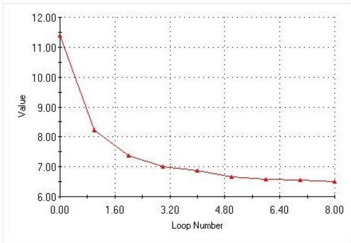
Slika 7.1 Dijagram konvergencije
