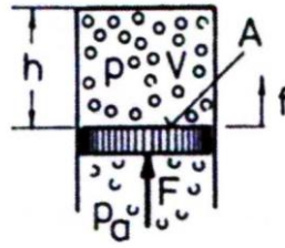
Slika 4.7 Skica pneumatske opruge
