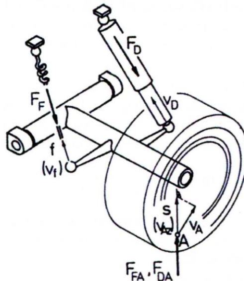
Slika 4.1 Neovješeni ovjes sa zavojnom oprugom i teleskopskim prigušivačem
