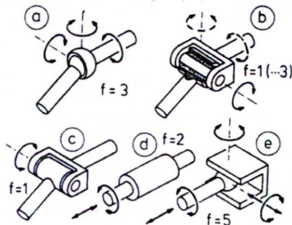
Slika 2.2 Izvedbe zglobova [1]
