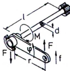
Slika 4.4 Torzijske opruge
