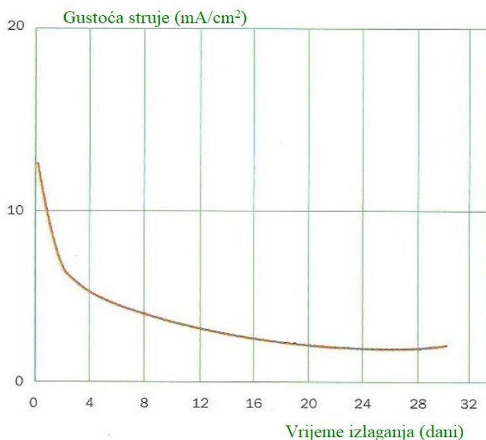
Slika 10. Katodna gustoća struje u vremenu za čelik Ultra 254 SMO (EN 1.4547) u 3% otopini natrijevog klorida pri 20 °C, pri polarizaciji od -300 mV [5]
