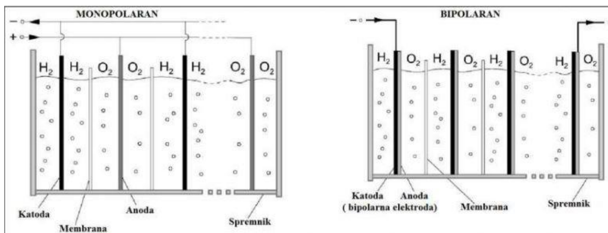
Slika 2. Monopolarna i bipolarna izvedba elektrolizatora [6]
