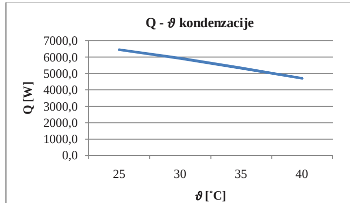
Slika 11 – Q\theta dijagram kondenzacije
