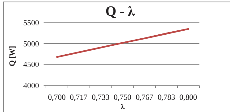
Slika 9 – Q\lambda dijagram
