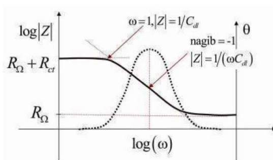
Slika 34. Bodeov dijagram [10]
