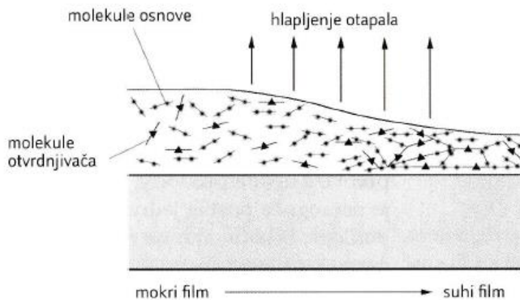
Slika 9. Dvokomponentno sušenje [8]
