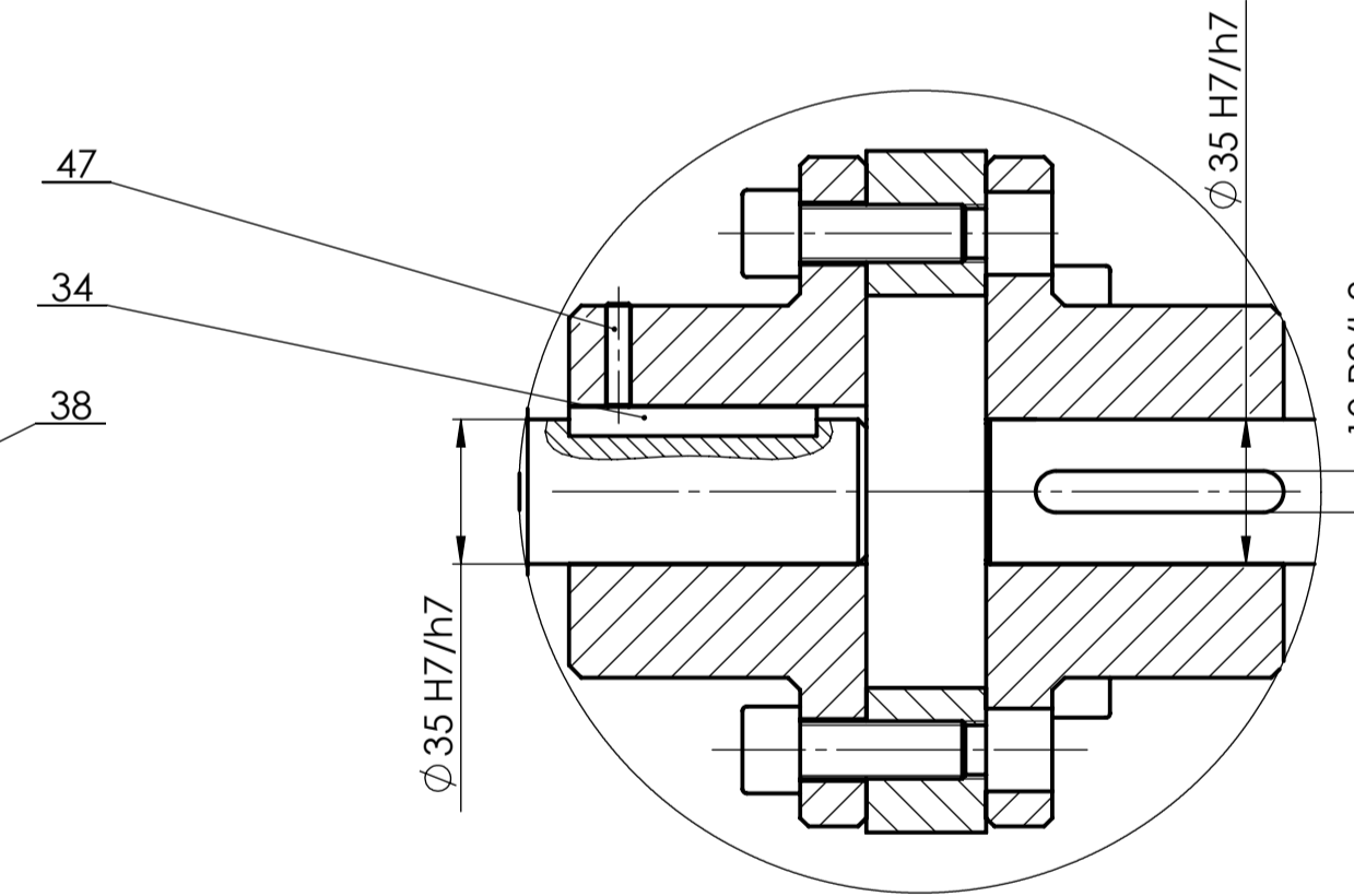
DETALJ G 1:1
