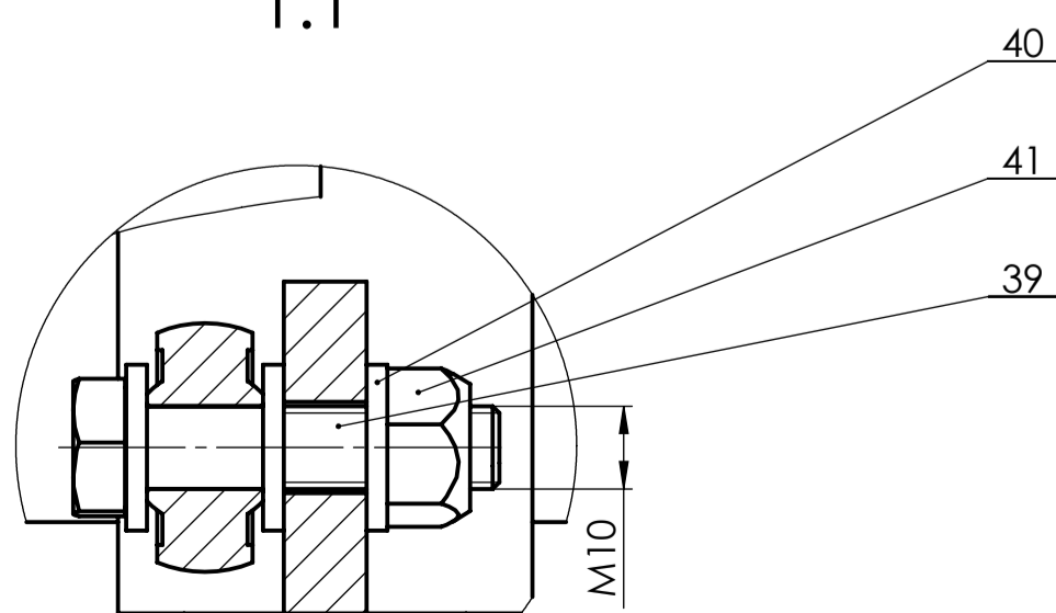
DETALJ D 1:1
