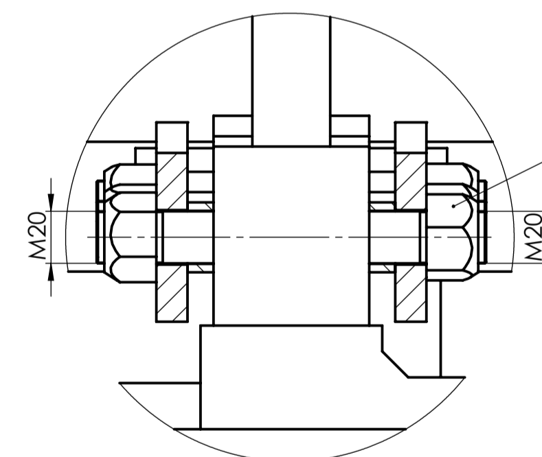
DETALJ C 1:2
