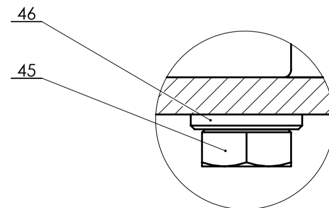
DETALJ E 1:1
