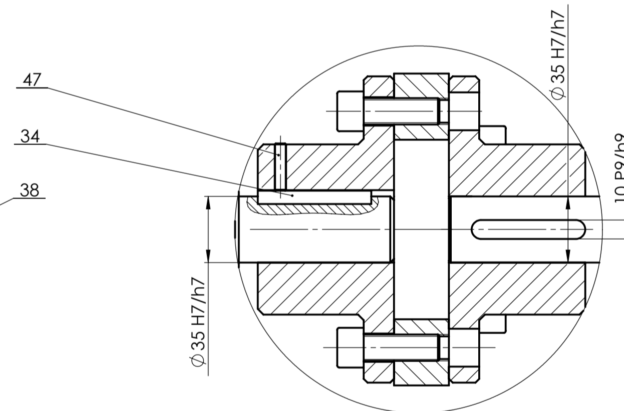
DETALJ G 1:1
