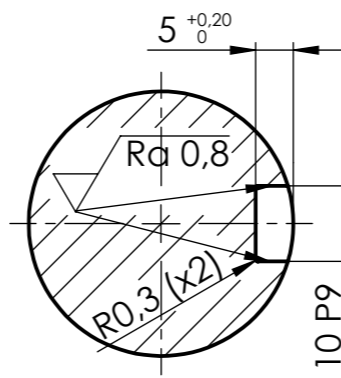
C-C 1:1
