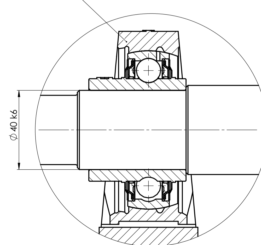
DETALJ G 1:1
