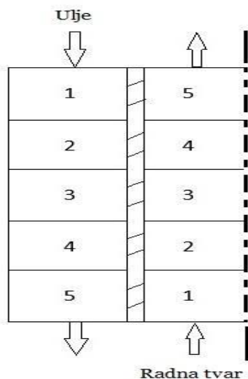
Slika 9. Segmentirani isparivač
