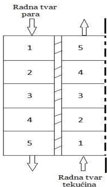
Slika 10. Segmentirani regenerator
