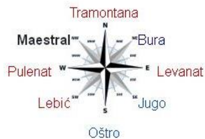
Slika 1-3 Vjetrovi Jadrana
