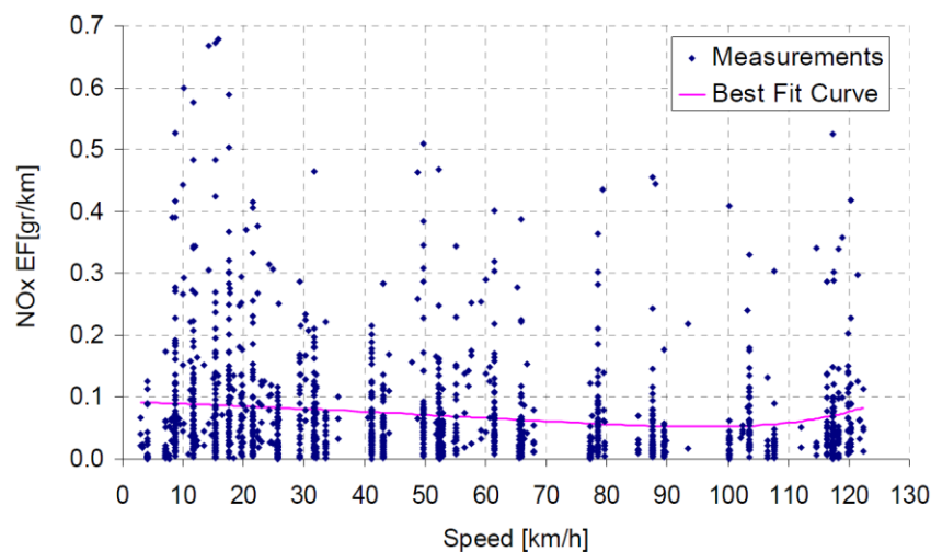
Slika 4.44. Primjer varijabilnosti rezultata mjerenja emisijskih faktora. Izvor: Kouridis et al. (2010) [100]
