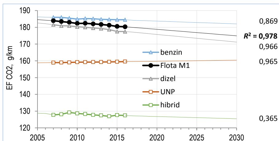
Slika 5.11. Emisijski faktori CO 2 hrvatske flote M1 po pojedinim vrstama goriva (od 2007. do 2016. podaci izračunati programom COPERT 5, ostalo linearna regresija)
