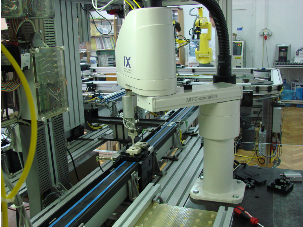
Slika 6.19 Umetanje krivuljne osovinice pomoću SCARA robota.
