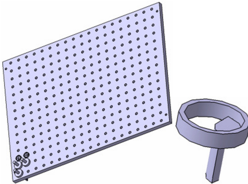
Slika 5.5. Paleta izvedena sa ulošcima za orijentiranje osovina i prikaz pojedinog uložka.
