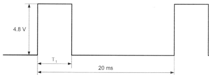
Slika 2. Prikaz upravljačkih impulsa
