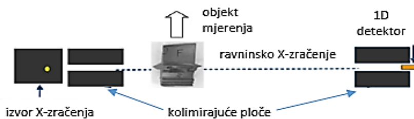
Slika 6 Princip rada linijskog CT uređaja [3]
