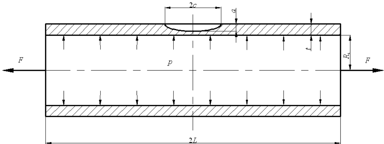
Slika 5.1. Cijev s polueliptičnom pukotinom opterećena unutarnjim tlakom
