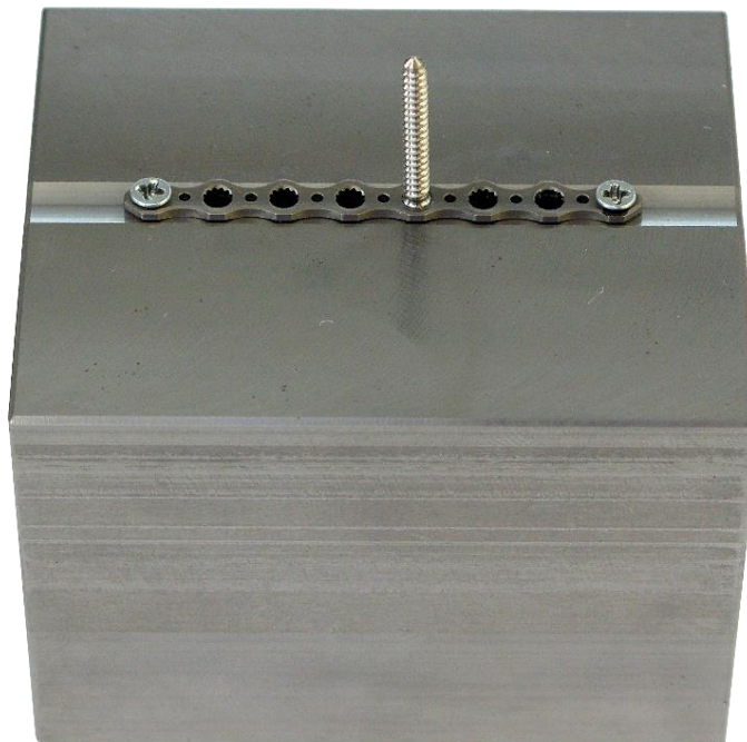
Slika 42. Pločica sa zaključanim vijkom pričvršćena na postolje
