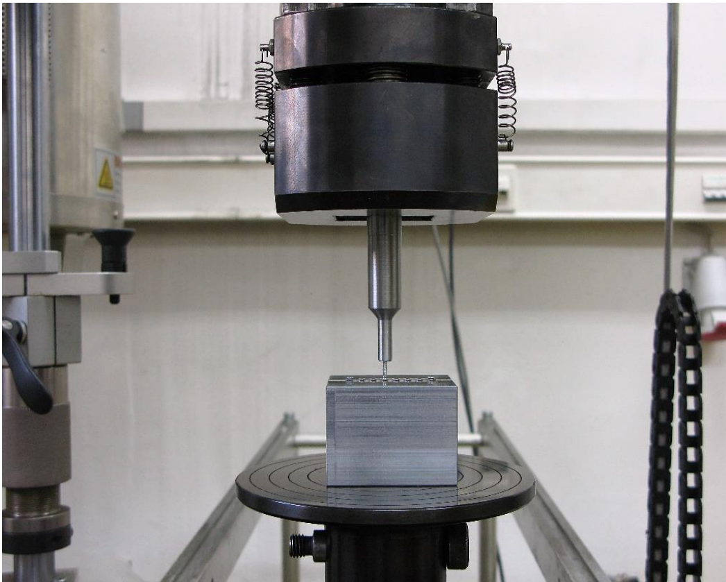
Slika 43. Eksperimentalni postav za test istiskivanja
