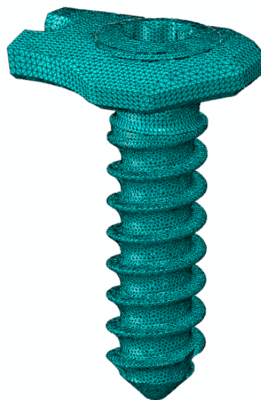
Slika 34. Računalni model kontrolnog zaključavanja: a) položaj vijka 0^\circ u odnosu na pločicu i b) generirana mreža konačnih elemenata
