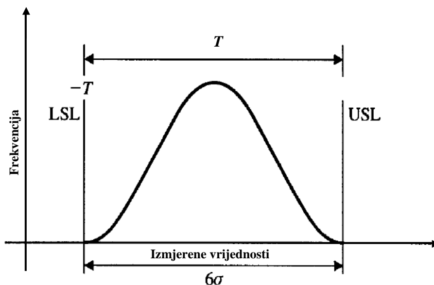
Slika 9. Sposobnost procesa [6]
