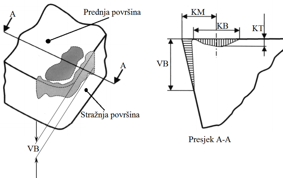
Slika 6. Parametri trošenja oštrice reznog alata [19]
