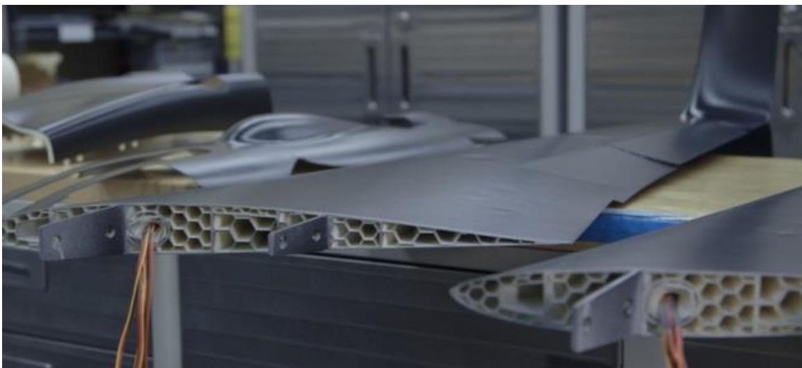
Slika 8 Krilo bespilotne letjelice Aurora Flight Sciences [8]
