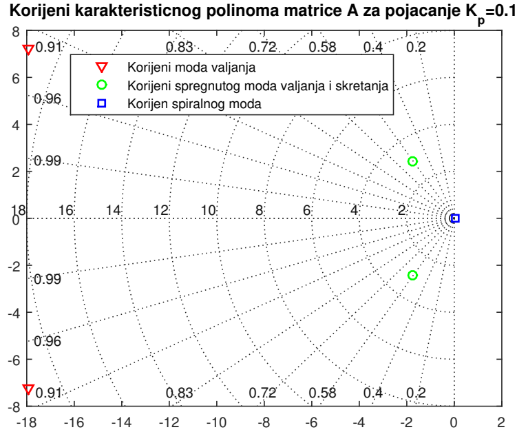
Slika 6.3: Korijeni karakterističnog polinoma matrice \mathbf{A} za K_p = 0.1
