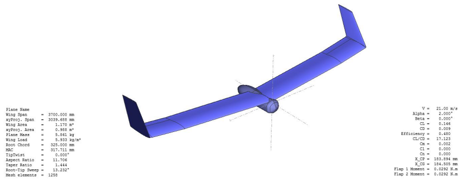
Slika 3.1: Geometrija unešena u XFLR i rezultati analize letjelice
