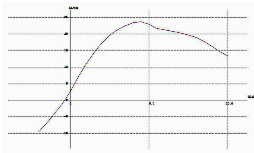
Slika 3.7: Finesa letjelice
