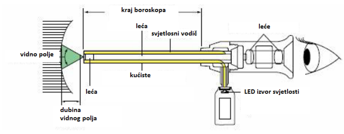
Slika 1. Presjek boroskopa [4]
