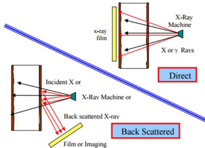
Slika 3.1. Usporedba sustava za snimanje tehnikom raspršenog zračenja i tehnike prozračivanja [7]
