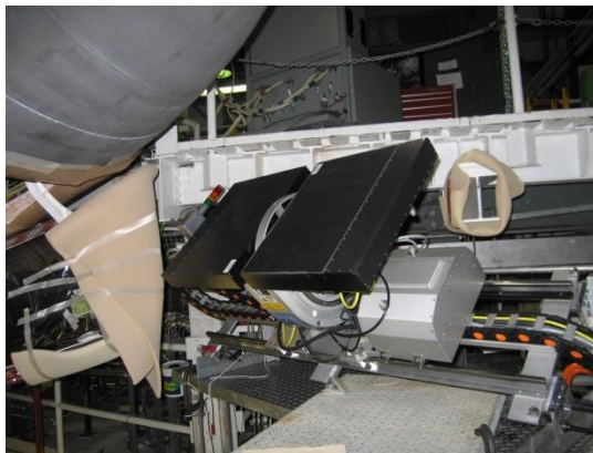
Slika 4.1. Uređaj za rendgensko snimanje tehnikom raspršenog zračenja [8]
