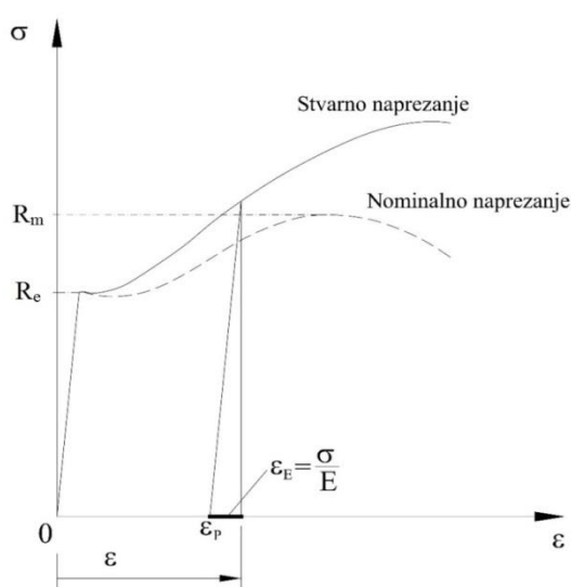
Slika 3.1. Kvalitativan prikaz krivulja nominalnog i stvarnog naprežanja duktilnog materijala, [1]
