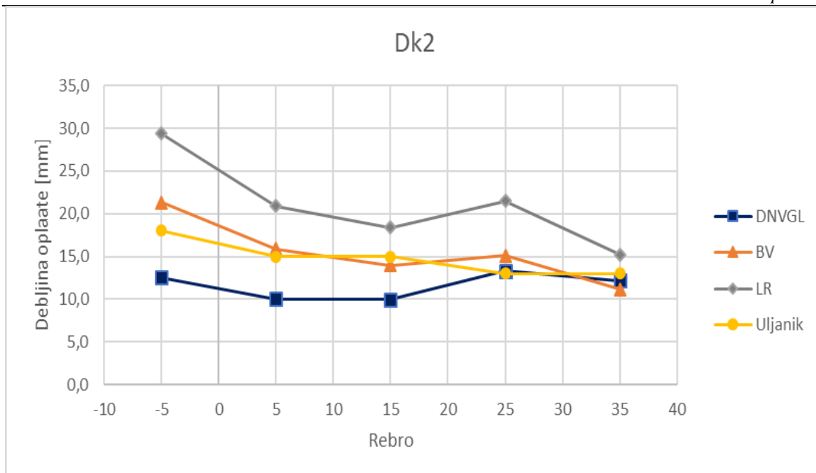
Slika 31. Raspored zahtijevanih debljina limova oplata na krmi na razini Dk 2
