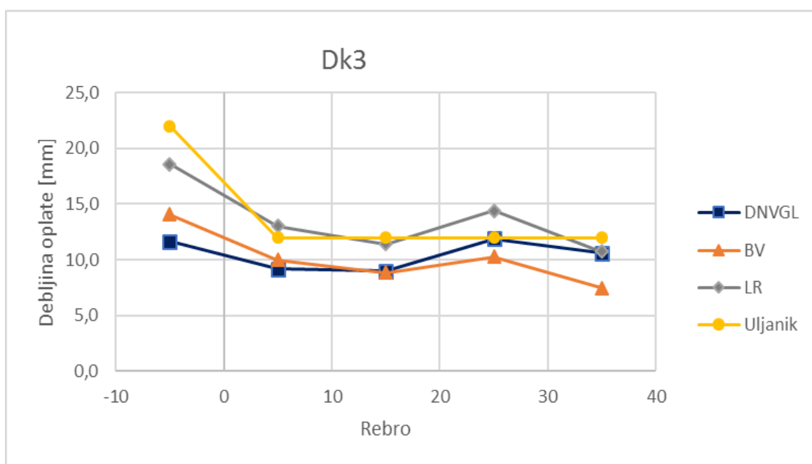
Slika 32. Raspored zahtijevanih debljina limova oplata na krmi na razini Dk 3
