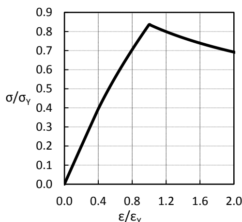
Slika 87. Primjer \sigma - \epsilon krivulje za globalno gredno – štapno izvicanje
