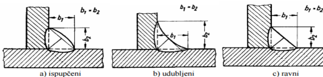
Slika 5. Kutni zavari
