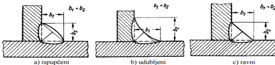
Slika 5. Kutni zavari
