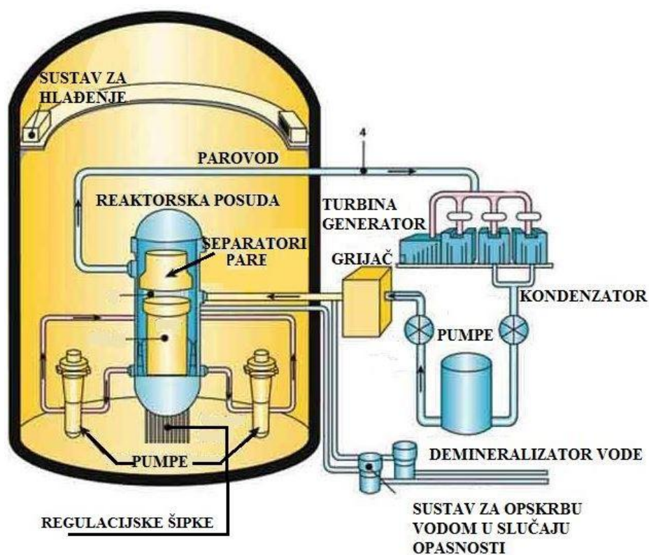
Slika 3.3 Kipući reaktor [10]
