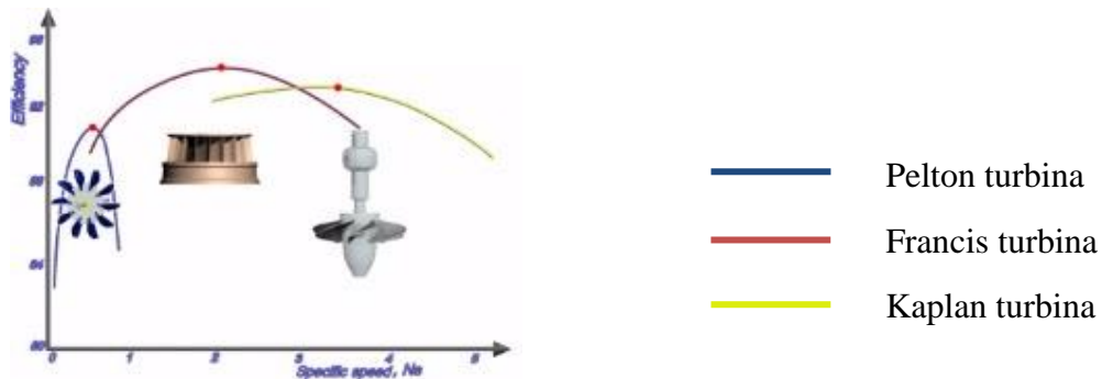
Slika 2. Iskoristivost Pelton, Francis i Kaplan turbine
