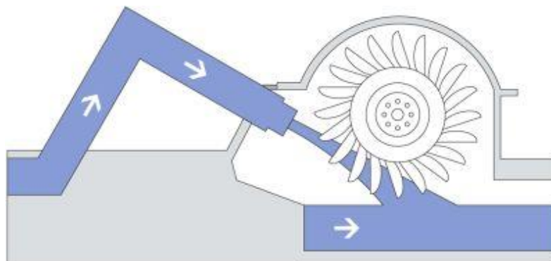
Slika 3. Princip rada Pelton turbine
