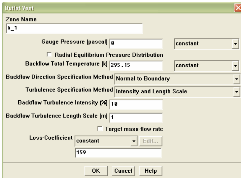
Slika 3.18. Rubni uvjet za otvore na trošilu
