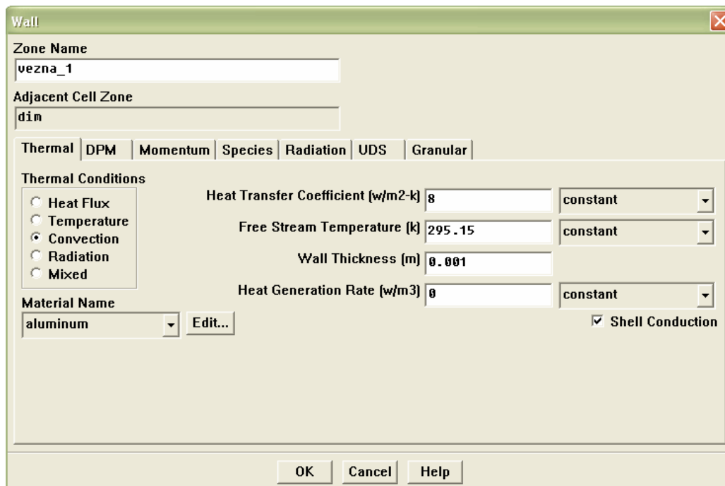
Slika 3.19. Rubni uvjet za vanjske površine vezne cijevi
