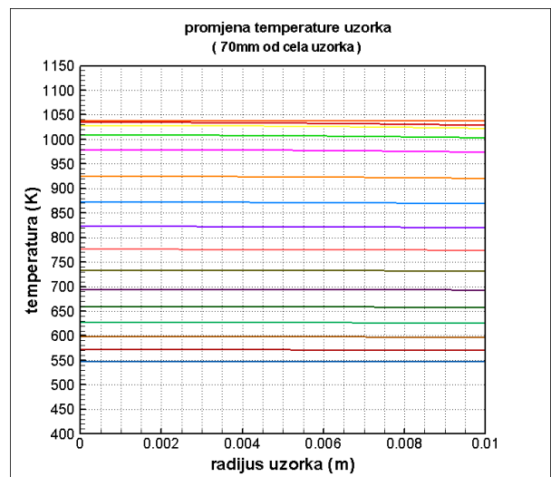
Slika 6.3 Promjena temperatura po poprečnom presjeku uzorka različito udaljenim od čela
