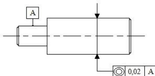
Slika 14. Tolerancija položaja
