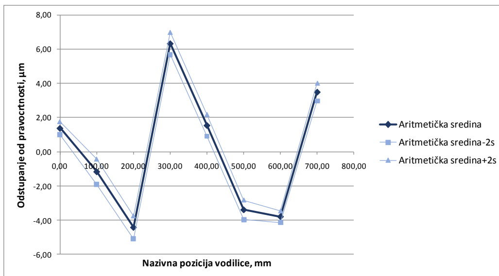
Slika 90. Aritmetičke sredine vertikalnih odstupanja od pravocrtnosti mjerenja u smjeru osi Y U idućoj tablici su, nakon daljnje analize, prikazani dobivena pogreška pravocrtnosti i odgovarajuće rasipanje rezultata.
