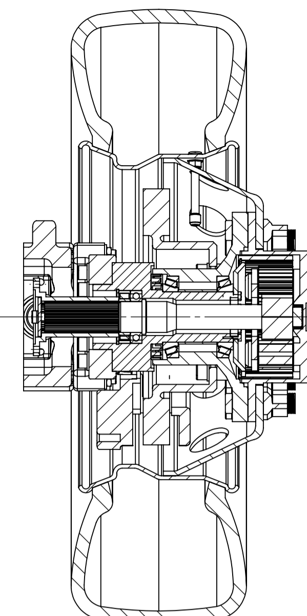
PRESJEK B-B MJERILO 1 : 5
