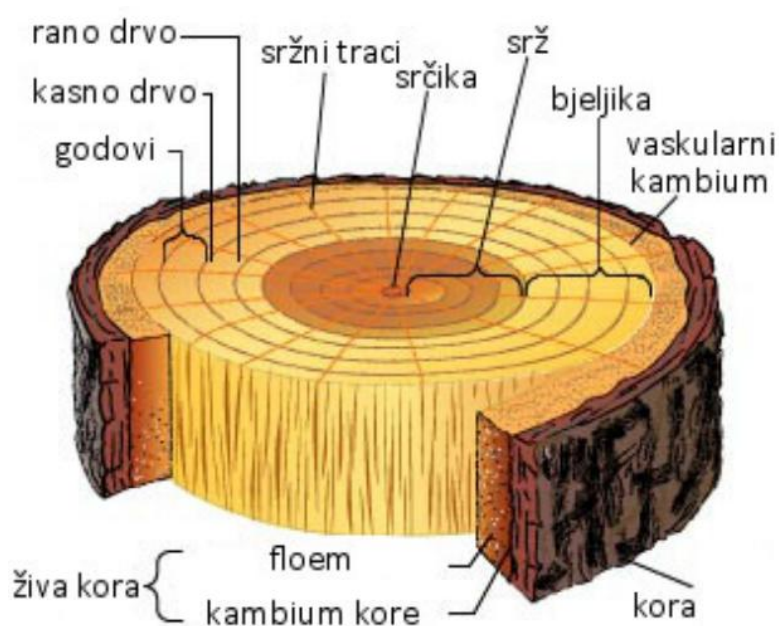
Slika 5. Makroskopski prikaz drva [8]
