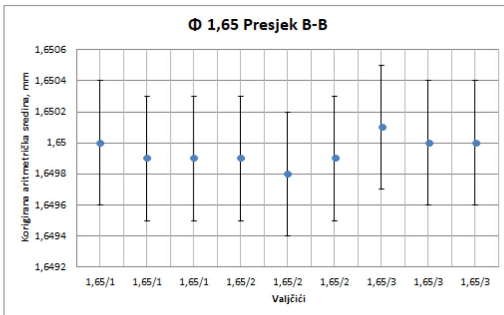
Slika 30. Vrijednosti sa pridruženom mjernom nesigurnosti valjčića \phi 1,65 u presjeku B-B
