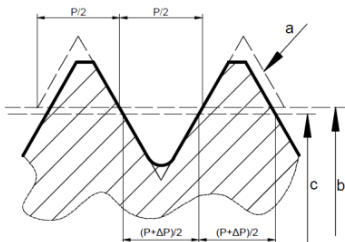
Slika 11. Profil navoja [10]
