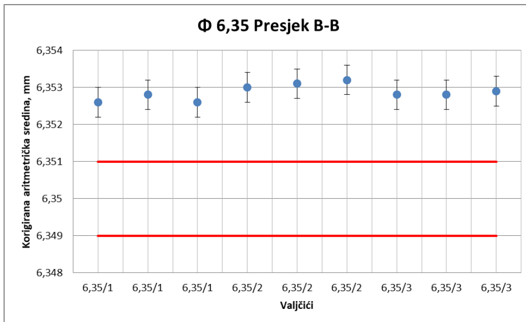
Slika 40. Prikaz valjčića \phi 6,35 u tolerancijskom polju na presjeku B-B
