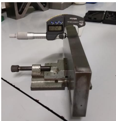
Slika 10. Prikaz mjerenja širine etalona br. 1 digitalnim mikrometrom
