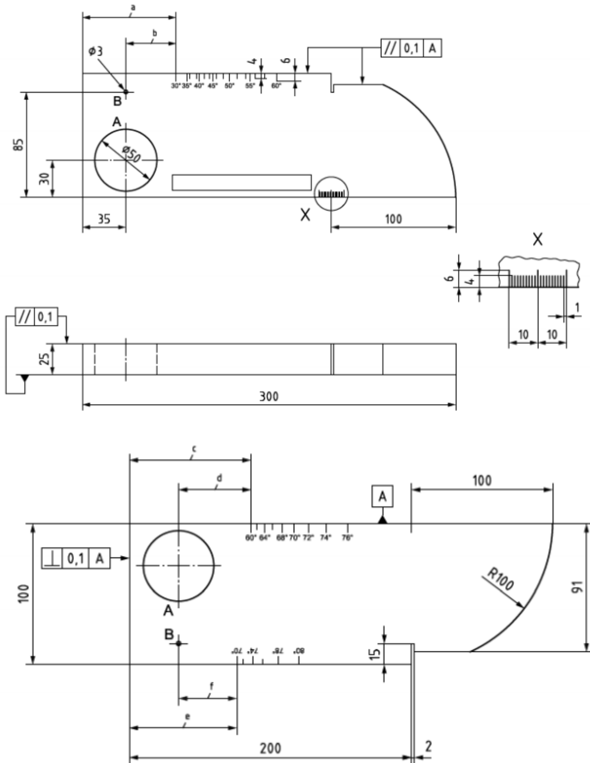
Slika 3. Dimenzije etalona br. 1
