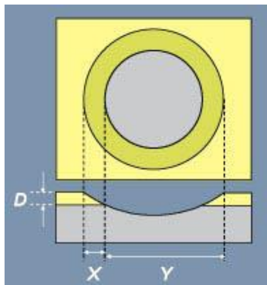
Slika 4.2 Shema kalotesta [8]
