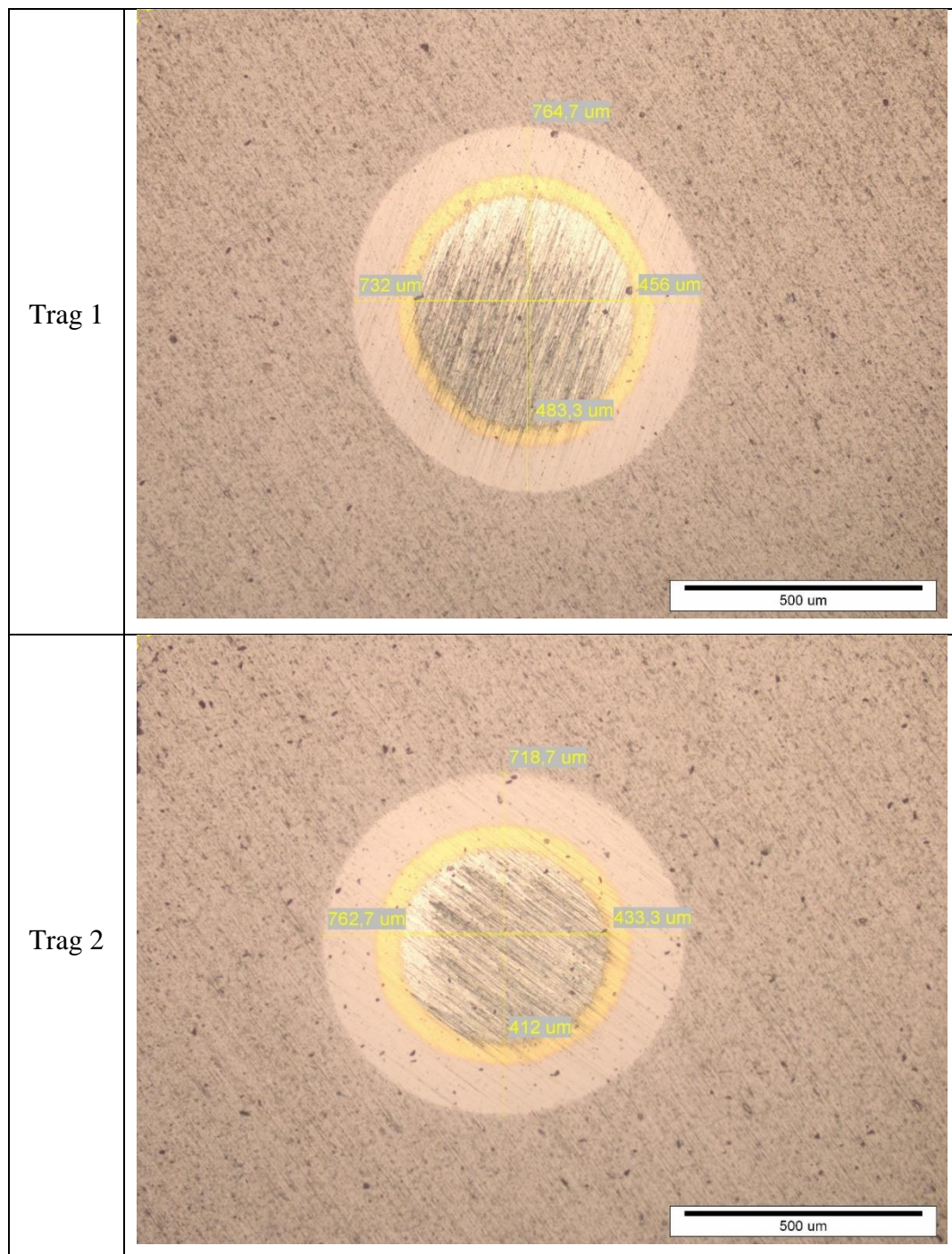
Prilog 17. Slike mjerenja debljine kalostestom za tragove 1, 2, 3 i 4.
