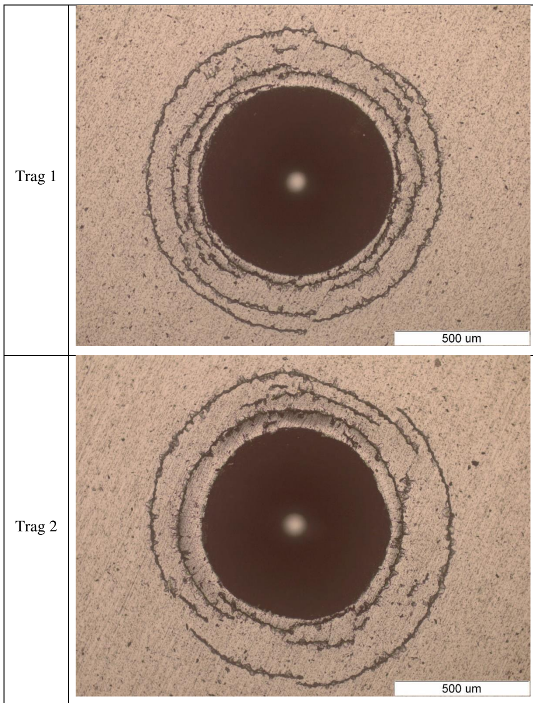
Prilog 18. Tragovi ispitivanja adhezivnosti prevlake po VDI testu.
