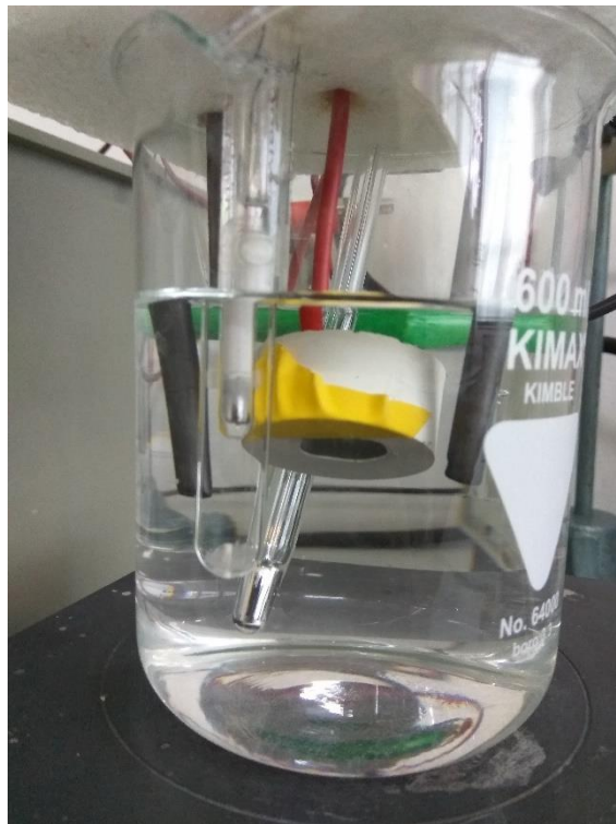
Slika 5.6 Raspored elektroda u elektrolitu
