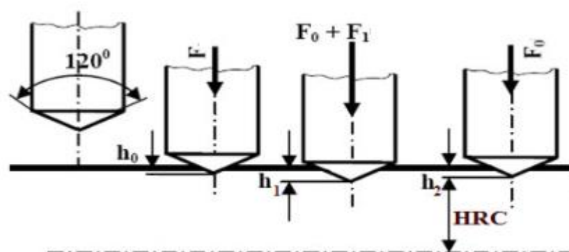
Slika 6. Ispitivanje tvrdoće Rockwellovom metodom s indentorom u obliku stošca [9]
