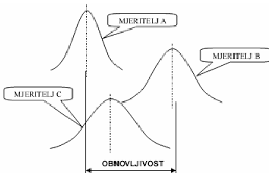
Slika 2. Obnovljivost rezultata [6]
