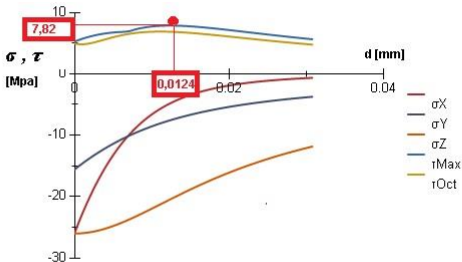
Sl. 25 Raspored naprežanja obzirom na udaljenost od površine
