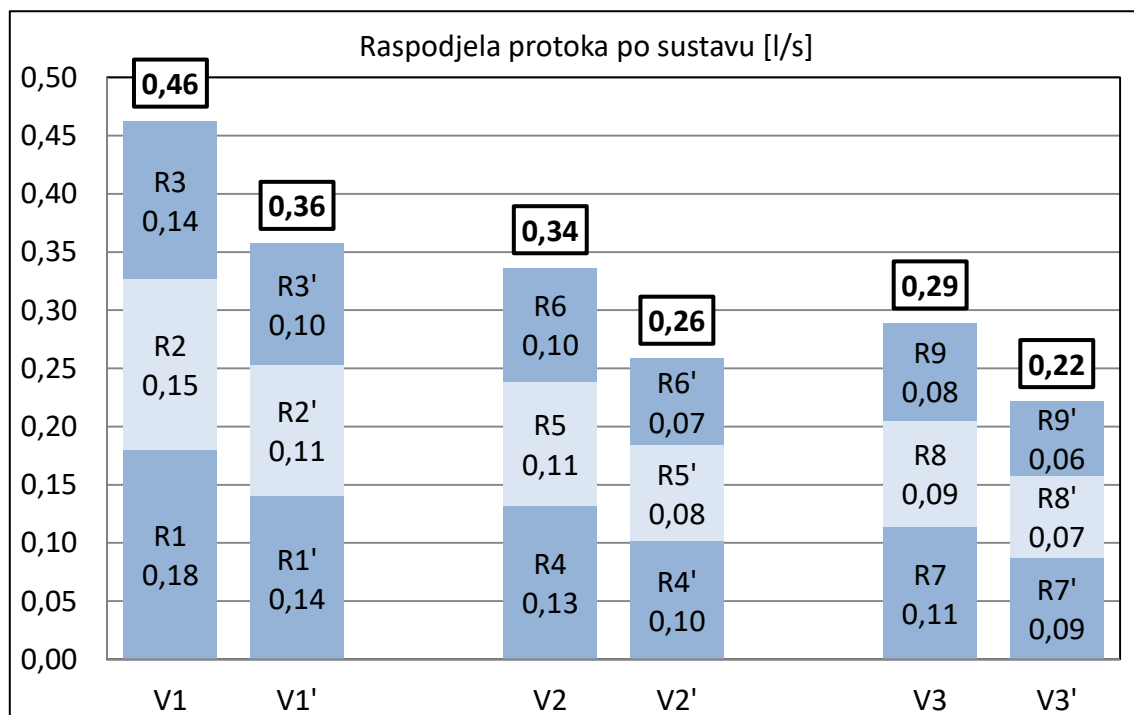
Slika 5.3. Usporedba raspodjele protoka pri projektним uvjetima
