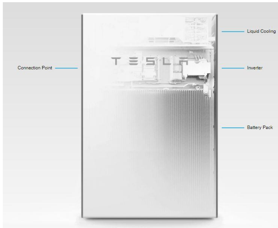
Slika 18. Baterija proizvođača Tesla [16]
