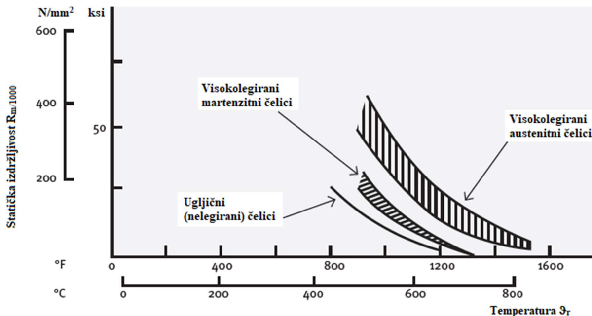
Slika 7. Orijentacijski prikaz ovisnosti statičke izdržljivosti o radnoj temperaturi za nelegirane, visokolegirane martenzitne i visokolegirane austenitne čelike [8]
