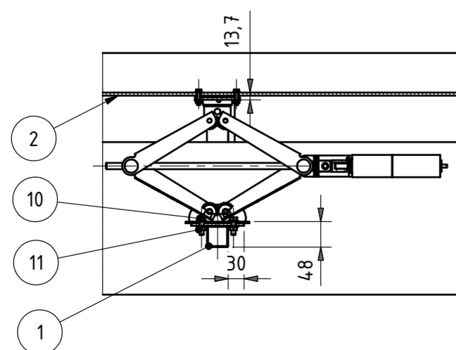
Presjek C-C M 1:10
