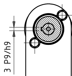
Presjek B-B M1:2
