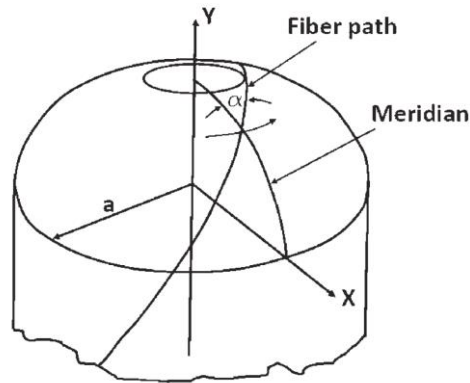
Slika 10. Geodetski put
