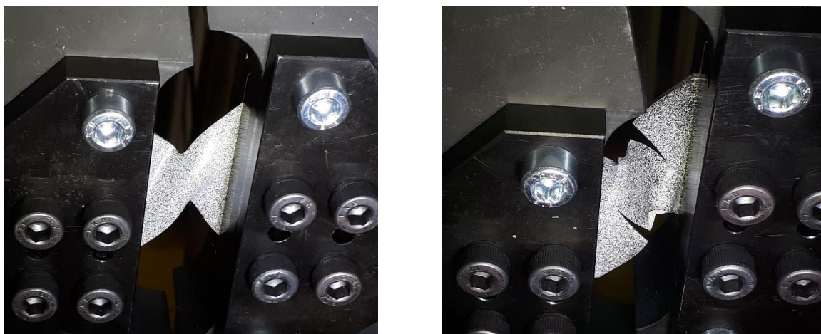
a) b) Slika 7.3. Prikaz izvijanja uzoraka debljine: a) 1 mm, b) 2 mm
