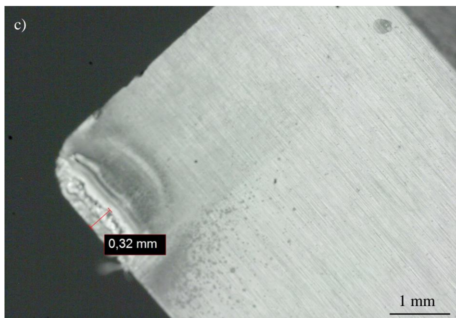
Slika 45. Trošenje prednje površine rezne pločice:
