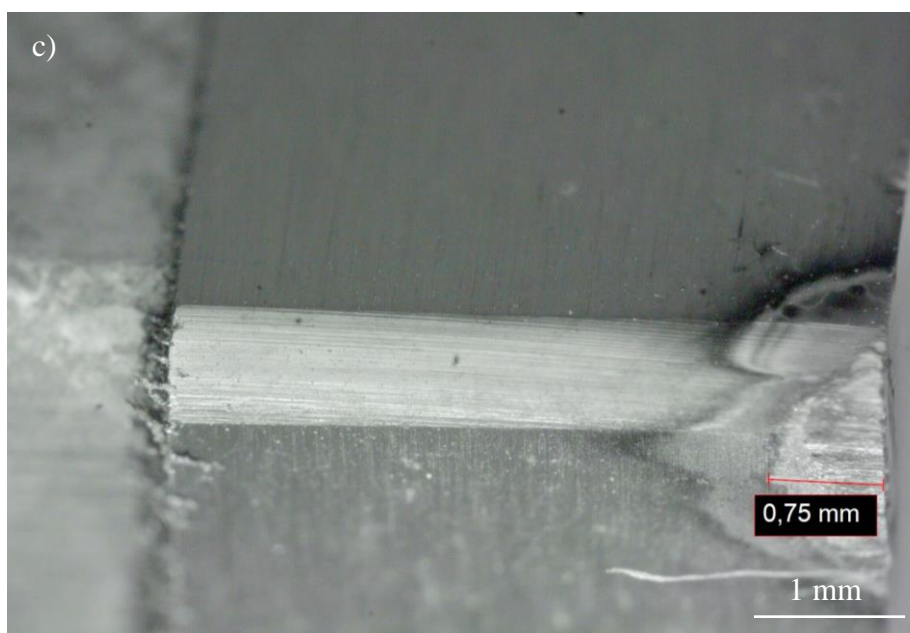
Slika 43. Trošenje stražnje površine rezne pločice:
