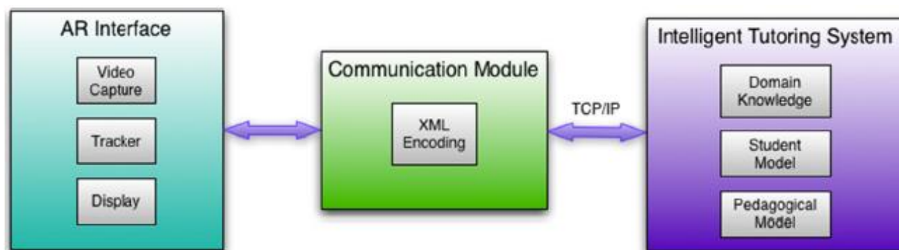
Slika 7.1. Struktura MATa [35]
