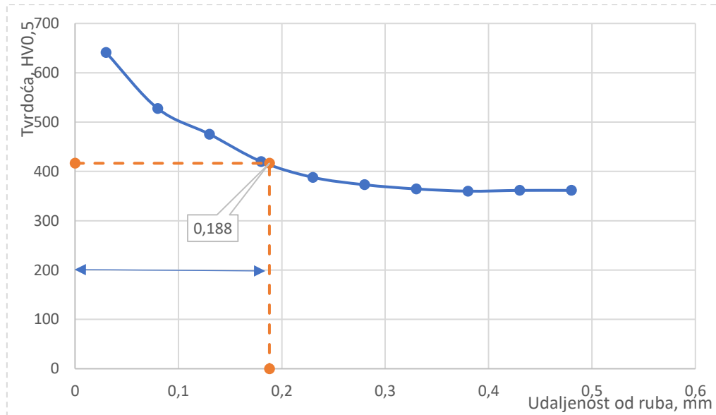
Slika 42. . Efektivna dubina nitriranja prstena nitriranog u plinu
