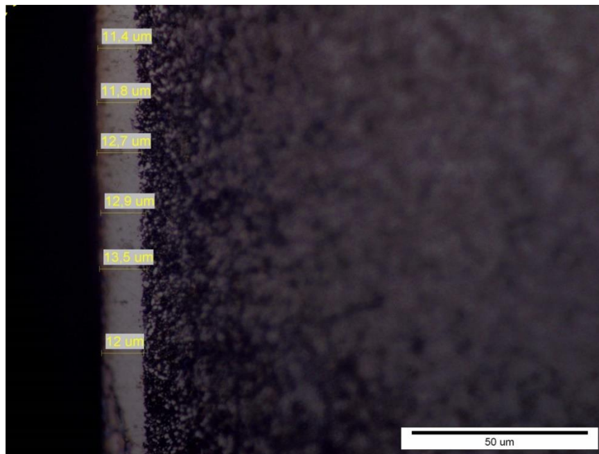
Slika 38. Debljina zone spojeva prstena nitriranog u solnoj kupci TENIFER povećanje 1000X
