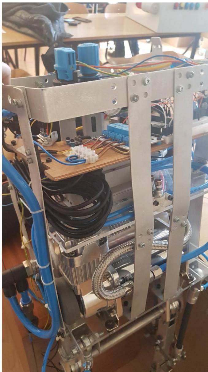
Slika 13. Izrađen trup robota
