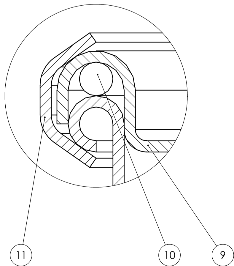
B-B (5:1)
