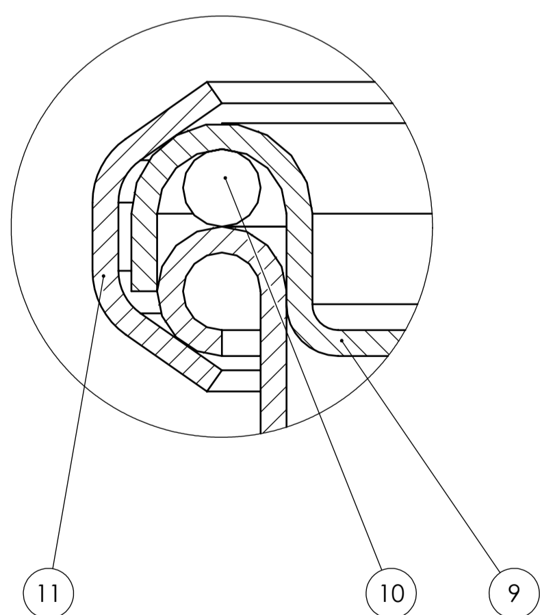
B-B(5:1)
