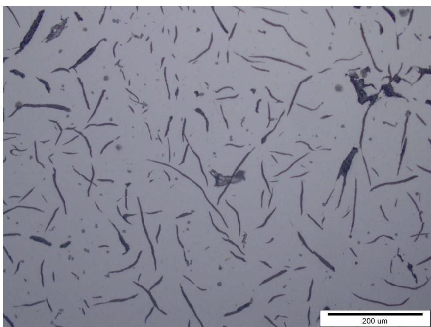
Slika 54. Mikrostruktura polirane površine kočionog diska 2 pri povećanju od 200x
