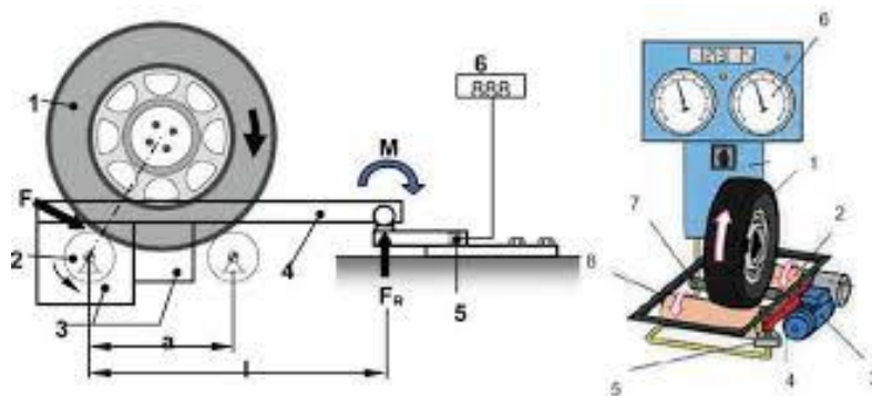
Slika 3. Shema valjaka za ispitivanje kočnica [3]
